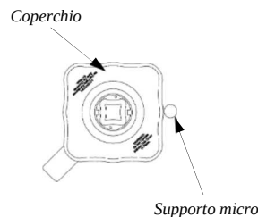
FIG.n°7 - Posizionamento coperchio bicchiere
