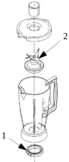
FIG.n°9 - Rimozione del porta coltelli
