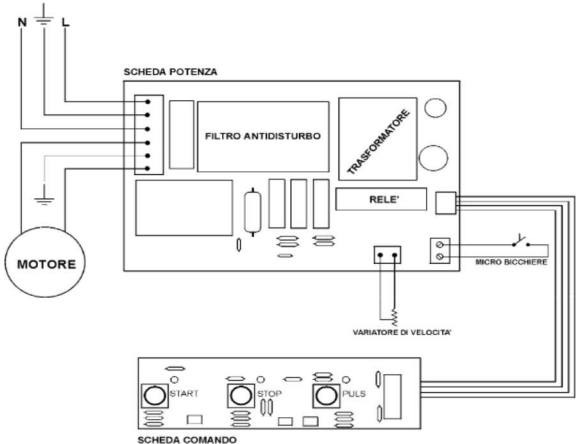
FIG. n°5 - Schema elettrico
